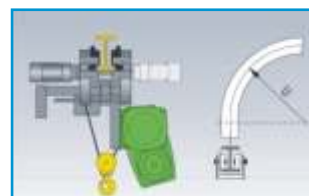
Talha com trole baixa altura para trechos retos "KE"
